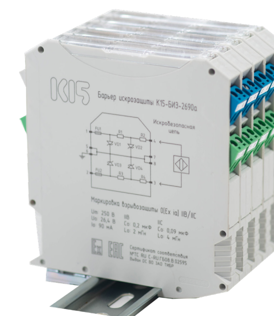
Барьеры искрозащиты
